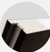
skrzydło stalowe z wzmocnieniem drewnianym i wypełnieniem z wełny mineralnej
