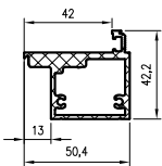
Profil DRE pre bezfalcové dvere otvárané von
