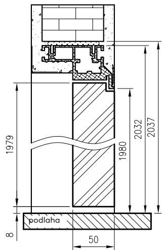
Vertikálny prierez 50mm dverí s obráteným falcem - otváranie dovnútra
