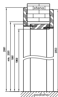
Vertikálna časť nastaviteľného tunela s uhl. T80
