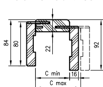
Prierez TUN s uhl. T63
