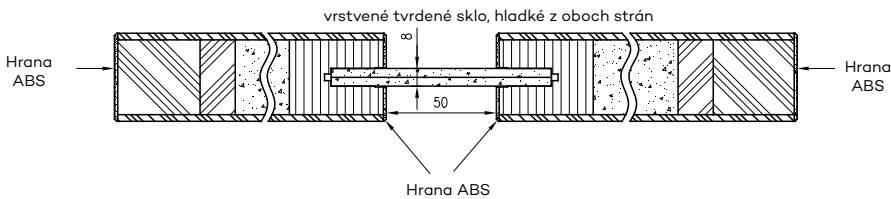
Vodorovný prierez bezfalcových dverí VETRO E
