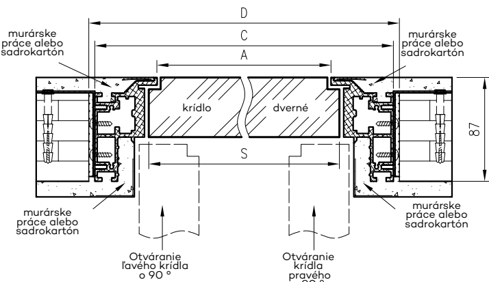
Priečny prierez 50mm dverí s obráteným falcem - otváranie dovnútra
